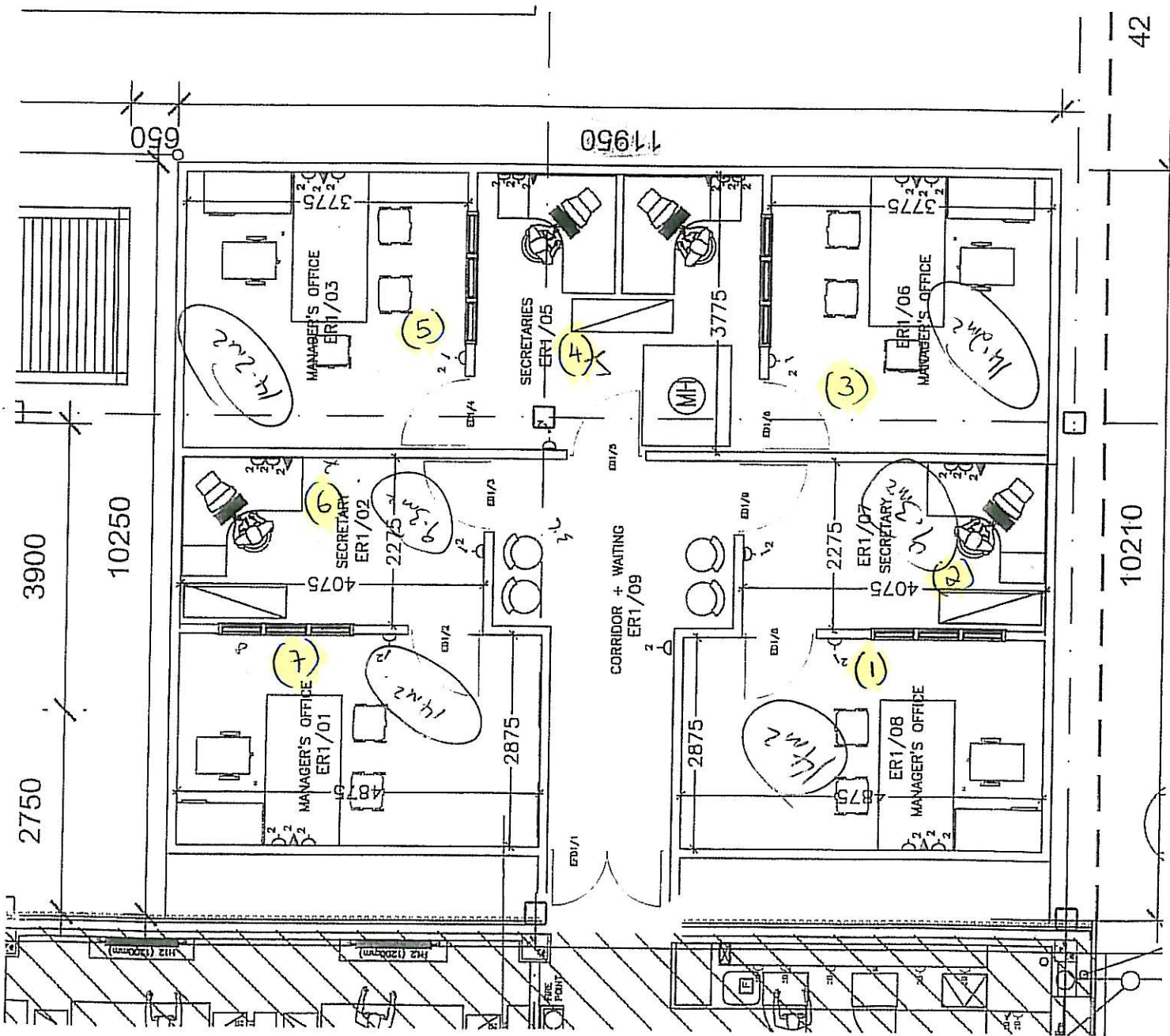
Portacabin 1
